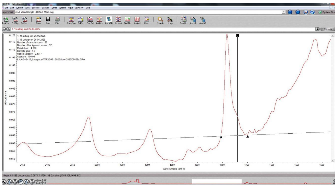
Figur 5. Eksempel på bestemmelse af 1720\text{ cm}^{-1} tophøjde på materialet efter ældning (aflæst til 0.0122)
