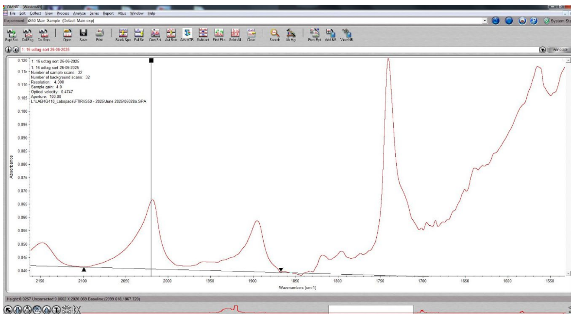
Figur 4. Eksempel på bestemmelse af 2020\text{ cm}^{-1} tophøjde på materialet efter ældning (aflæst til 0.0257)
