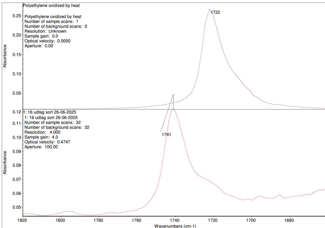
Figur 1. Øverste FTIR-spektrum viser, hvordan oxidativt nedbrudt polyethylen har et tydeligt carbonyl-signal omkring 1720 cm -1 . Nederste FTIR-spektrum viser, at den polyethylen der er anvendt til kilerne kun har et carbonylsignal ved 1720 cm -1 , der udgør en lille skulder. Carbonylsignalet, der topper omkring 1741 cm -1 anses at skyldes proceshjælpstoffer (fx antioxidanter).
