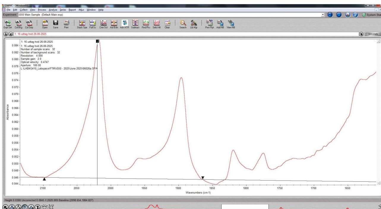
Figur 4. Eksempel på bestemmelse af 2020\text{ cm}^{-1} tophøjde på materialet efter ældning (aflæst til 0.0388)
