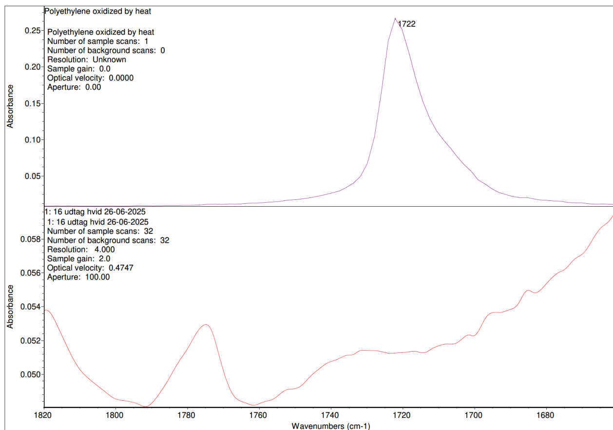
Figur 1. Øverste FTIR-spektrum viser, hvordan oxidativt nedbrudt polyethylen har et tydeligt carbonyl-signal omkring 1720 cm -1 . Nederste FTIR-spektrum viser intet tilsvarende carbonylsignal.
