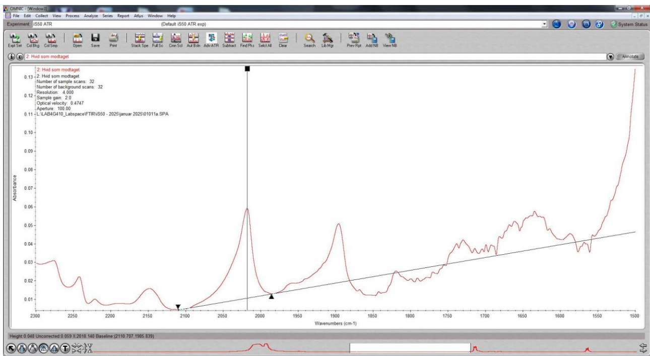
Figur 2. Eksempel på bestemmelse af 2020 cm -1 tophøjde på materialet før ældning (her aflæst (0.048))
