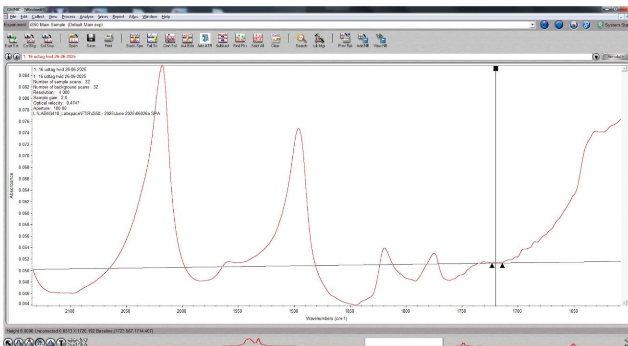
Figur 5. Eksempel på bestemmelse af 1720\text{ cm}^{-1} tophøjde på materialet efter ældning (aflæst til 0.0000)
