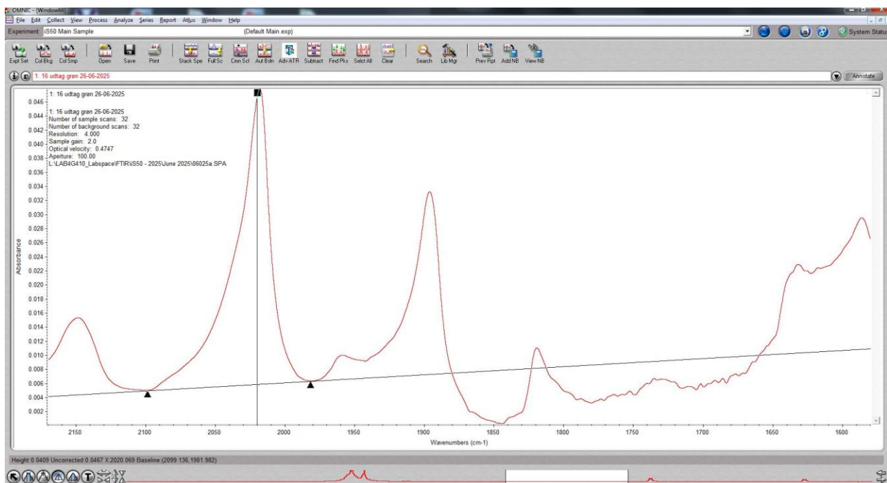
Figur 4. Eksempel på bestemmelse af 2020 cm -1 tophøjde på materialet efter ældning (aflæst til 0.0409)
