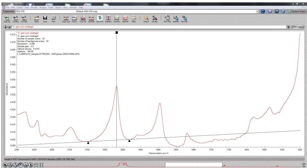
Figur 2. Eksempel på bestemmelse af 2020\text{ cm}^{-1} tophøjde på materialet før ældning (her aflæst (0.0357))
