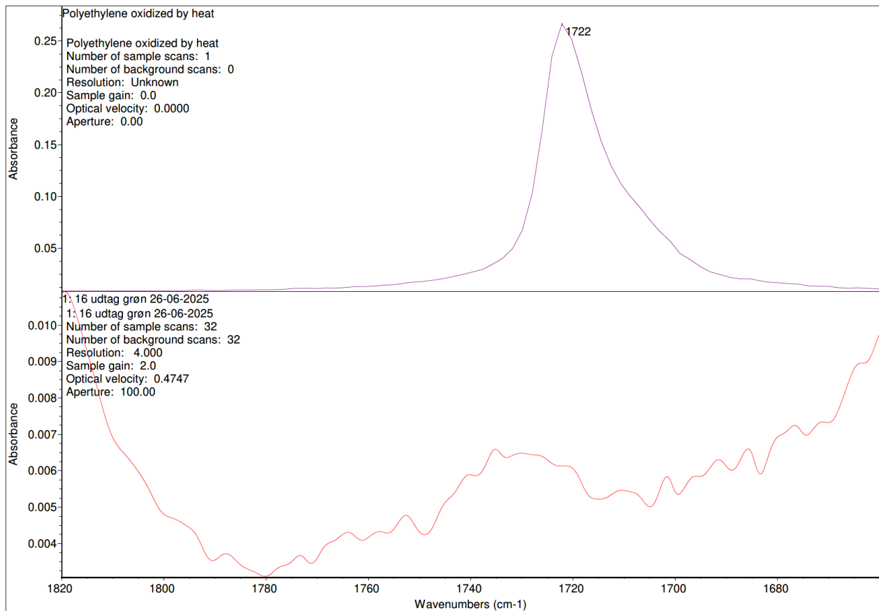
Figur 1. Øverste FTIR-spektrum viser, hvordan oxidativt nedbrudt polyethylen har et tydeligt carbonyl-signal omkring 1720\text{ cm}^{-1} . Nederste FTIR-spektrum viser et meget lille carbonylsignal.
