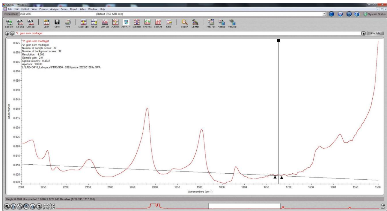
Figur 3. Eksempel på bestemmelse af 1720 cm -1 tophøjde før ældning (her aflæst til 0.0034)
