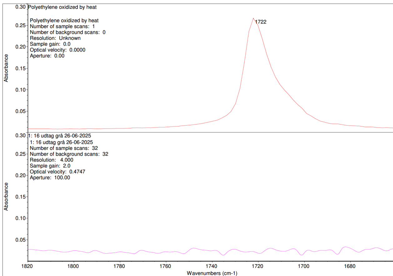
Figur 1. Øverste FTIR-spektrum viser, hvordan oxidativt nedbrudt polyethylen har et tydeligt carbonyl-signal omkring 1720 cm -1 . Nederste FTIR-spektrum viser ingen carbonylsignal.
