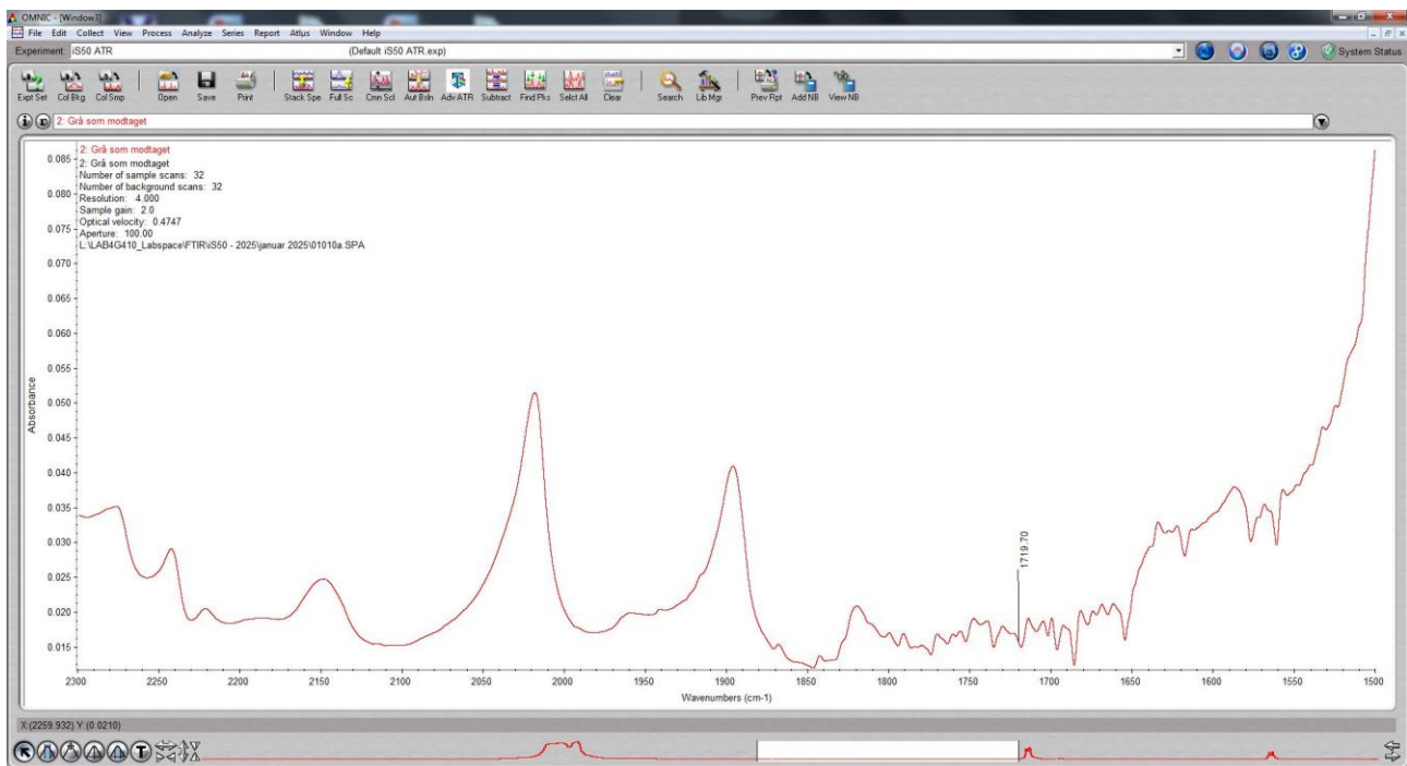
Figur 3. Eksempel på bestemmelse af 1720\text{ cm}^{-1} tophøjde før ældning (her aflæst til 0)
