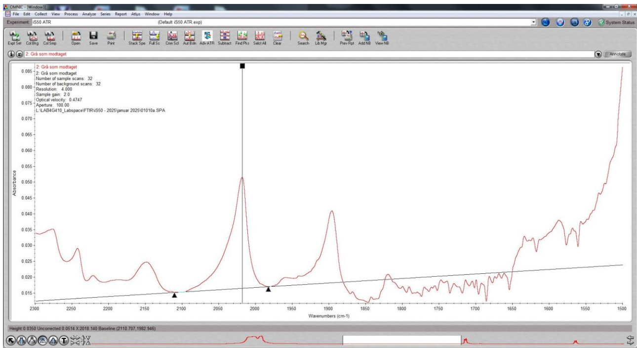
Figur 2. Eksempel på bestemmelse af 2020\text{ cm}^{-1} tophøjde på materialet før ældning (her aflæst (0.0350))
