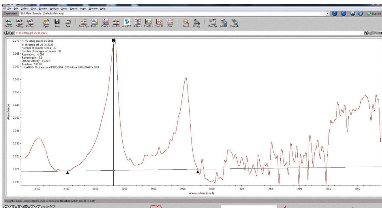
Figur 4. Eksempel på bestemmelse af 2020\text{ cm}^{-1} tophøjde på materialet efter ældning (aflæst til 0.0496)
